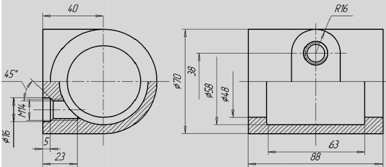
Корпус
