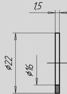
Прокладка
